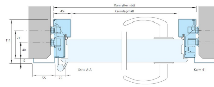
Skiss enkeldörr, snitt A-A.
